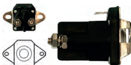
231525 Solenoid 12 V, 80 Amp, B+ 1/4"-20, Kl. 15a 10-24 UNC, Kl. 50 10-24 UNC, Total length 66.45, Height/B+ 18.00, Coil bolt 1/4"-20, Coil bolt 2 18.00, No./terminals 4 Insulated return.
