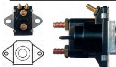
139857 Solenoid 12 V, B+ M8, Kl. 15a M4, Kl. 50 M4, OD 55.90, Total length 55.45, Height/B+ 10.70, Width/Kl. 15a 9.65, Width/kl. 50 9.30, Coil bolt M8, Coil bolt 2 10.65, No./terminals 4
