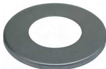
134271 Dp Cap ID 65.02, OD 66.90
