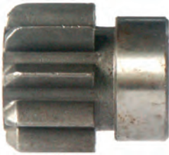
134197 # Dp Gear ID 11.65, OD 25.30, Height 27.85, No./teeth 9
