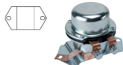
333018 Solenoid 24 V, 100 Amp, Kl. 50 M4, Total length 87.00, Height/B+ M8x1.25, Coil bolt M8x1.25, No./terminals 3
