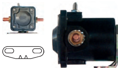
139860 Solenoid 12 V, Kl. 50 M5, OD 54.00, Total length 64.20, Height/B+ 13.25, Width/kl. 50 8.55, Coil bolt 2 13.55, No./terminals 3
