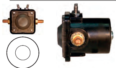
139859 Solenoid 12 V, B+ M8, Kl. 15a M5, Kl. 50 M5, OD 53.85, Total length 64.00, Height/B+ 12.30, Width/Kl. 15a 8.25, Width/kl. 50 8.50, Coil bolt M8, Coil bolt 2 12.15, No./terminals 4
