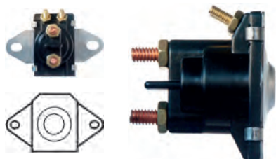
139856 Solenoid 12 V, B+ M8, Kl. 15a M4, Kl. 50 M4, OD 56.00, Total length 55.80, Height/B+ 10.55, Width/Kl. 15a 9.20, Width/kl. 50 9.75, Coil bolt M8, Coil bolt 2 10.40, No./terminals 4
