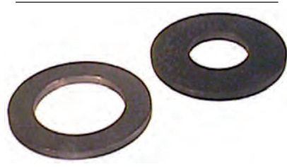
138649 Washer Kit Pkg. 10 Replacing: 182155 Servicing: D13E101TE, D13E105, D13E108TE, D13E111, D13E111TE, D13E116, D13E72, D13E73, D13E73TE, D13E74, D13E74TE, D13E78
