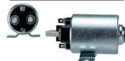
333008 Solenoid 24 V, 150 Amp, B+ M8, Kl. 50 6.30, OD 54.00, Total length 109.40, Height/B+ 15.00, Width/kl. 50 60.00, No./terminals 4
