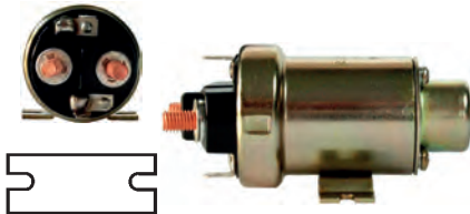
230964 Solenoid 24 V, 200 Amp, Intermittent load 800 Amp., B+ M8, Kl. 15a 6.30, Kl. 50 6.30, OD 44.90, OD/cover 47.45, Total length 115.50, Height/B+ 12.25, Width/kl. 15a 12.65, Width/kl. 50 11.70, Coil bolt M8, Coil bolt 2 12.00, Seconds 5, No./terminals 4
