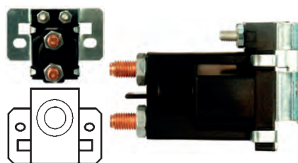
231527 Solenoid 12 V, 80 Amp, B+ 5/16"-24, Kl. 15a M5, Kl. 50 M5, OD 54.20, Total length 77.65, Height/B+ 11.55, Width/kl. 15a 7.00, Width/kl. 50 6.90, Coil bolt 5/16"-24, Coil bolt 2 11.45, No./terminals 4
