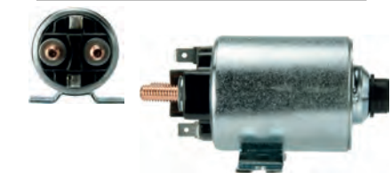
333017 Solenoid 24 V, 100 Amp, B+ M8, Kl. 15a 6.30, Kl. 50 6.30, OD 52.07, Total length 109.40, Height/B+ 15.00, Width/kl. 15a 30.00, No./terminals 4
