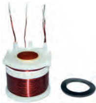
138937 Solenoid Coil 12 V, ID 21.00, OD 46.70
