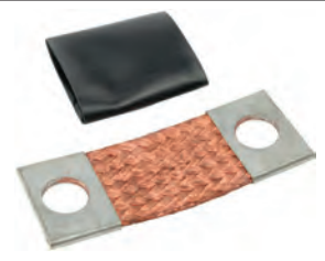
139535 Connection Replacing: 182159 Servicing: D13E100TE, D13E101TE, D13E104TE, D13E105, D13E107TE, D13E108TE, D13E109TE, D13E110TE, D13E111, D13E117TE, D13E118TE Mount. hole 12.60, Mount. hole 2 12.60, Total length 82.20
